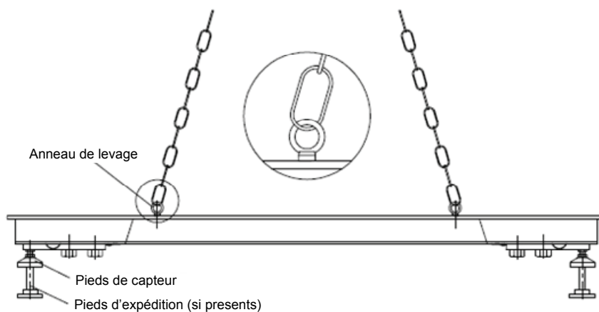
Figure 1 Méthodes de levage
