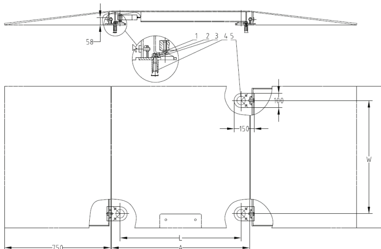
Figure 3. Installation de plaques de pieds et rampe optionnelles
