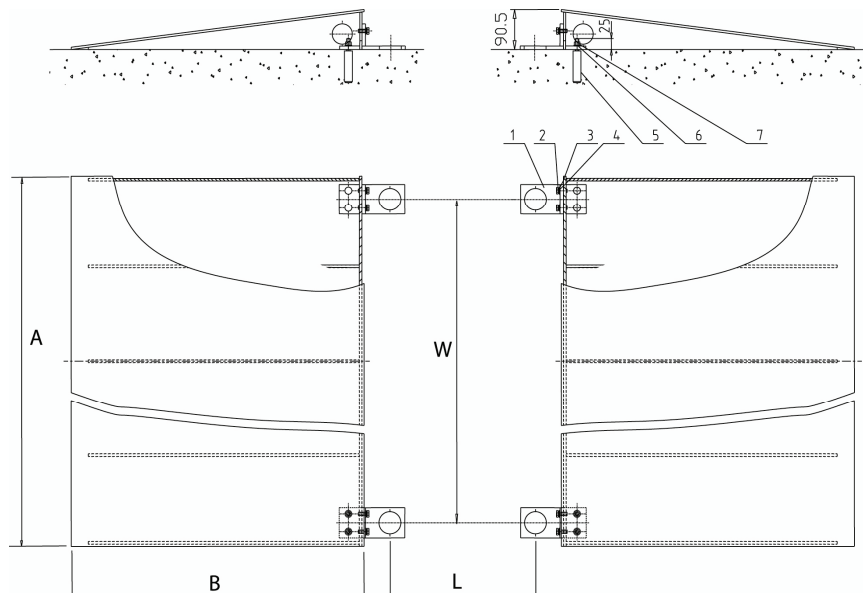
Figura 3. Installazione dei piedini di regolazione e delle rampe opzionali
