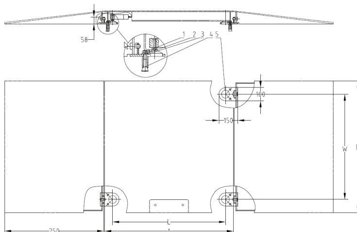
Figura 3. Instalación de placas para patas y rampas opcionales
